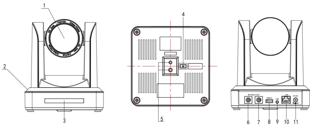
图 1.2 U2 型号接口
