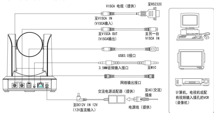
图 2.5 U3 外部接口示意图
