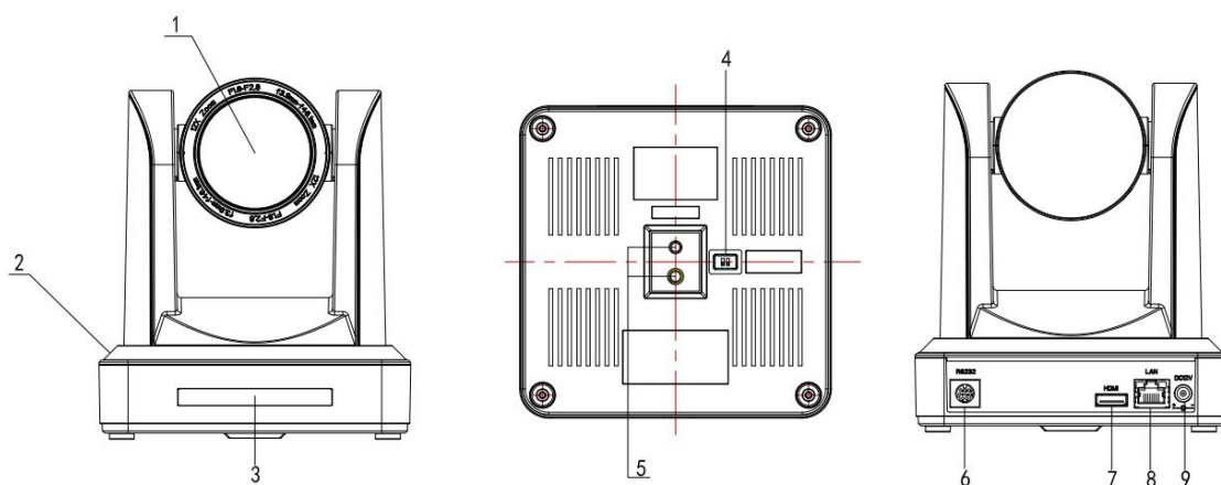
图 1.5 HM 型号接口
