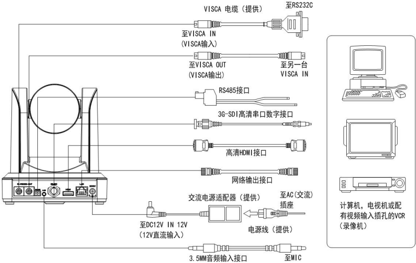
图 2.3 ST 外部接口示意图
