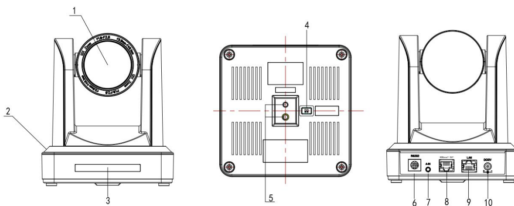
图 1.4 HD 型号接口
