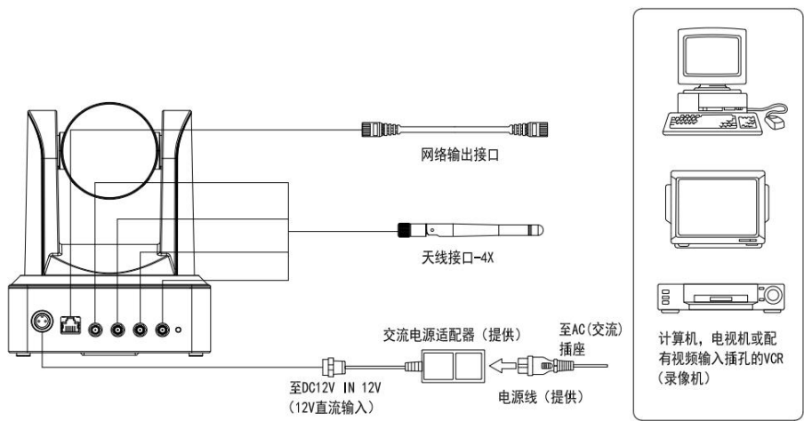
图 2.9 RF 外部接口示意图
