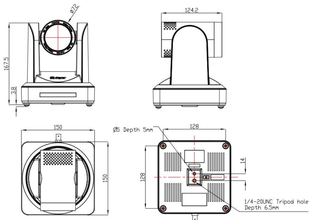
图 2.2 外型尺寸
