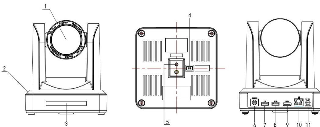
图 1.6 U2U3 型号接口
