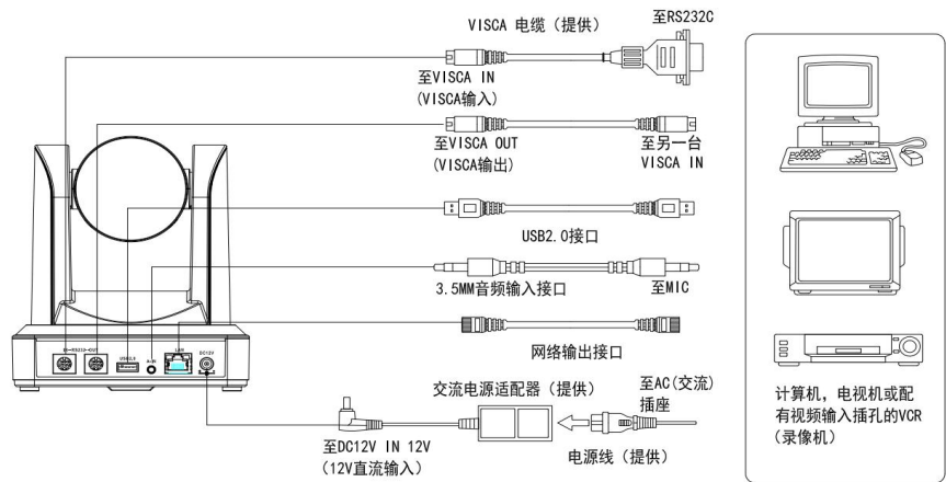
图 2.4 U2 外部接口示意图
