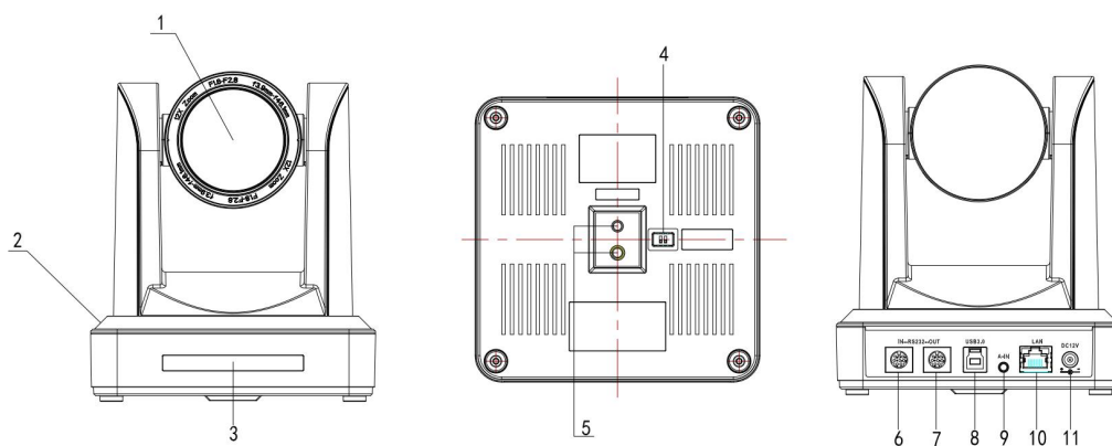
图 1.3 U3 型号接口
