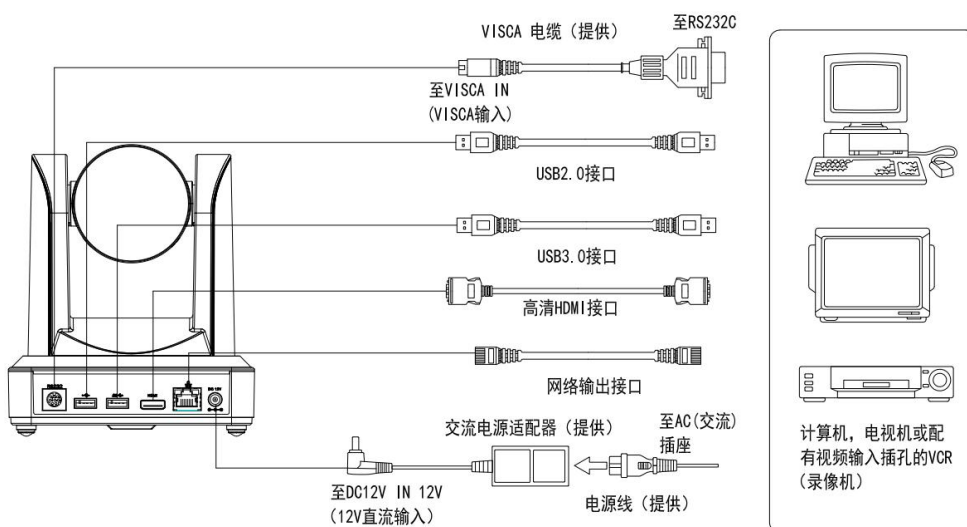
图 2.8 U2U3 外部接口示意图
