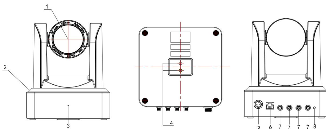
图 1.7 RF 型号接口
